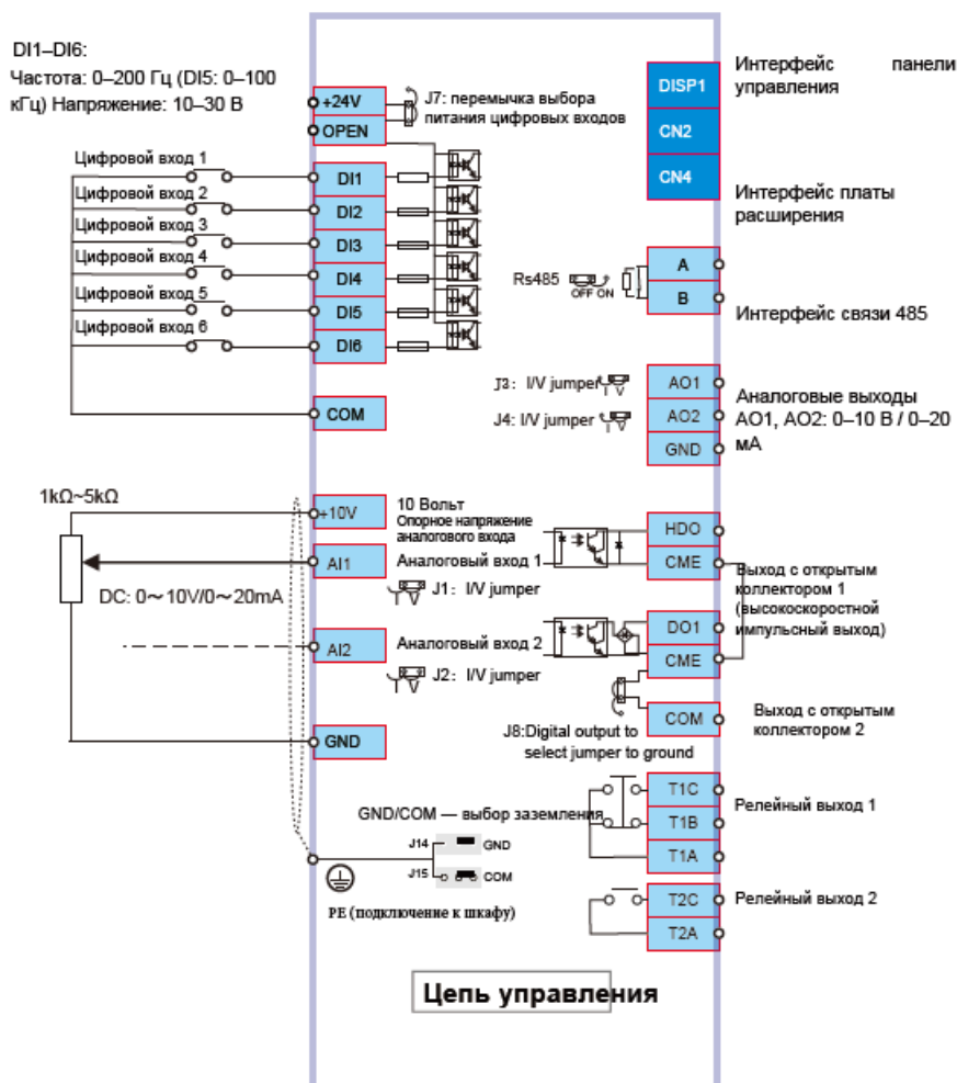
Рисунок 2 – Схема подключения для Sinovo SD600-4T-2.2G/4.0P
