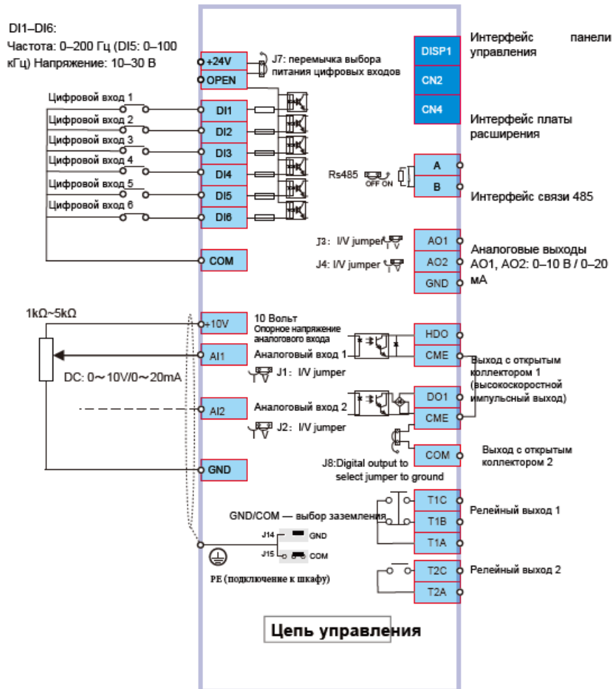
Рисунок 2 – Схема подключения
